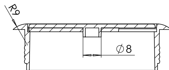
PRZEKRÓJ A-A
